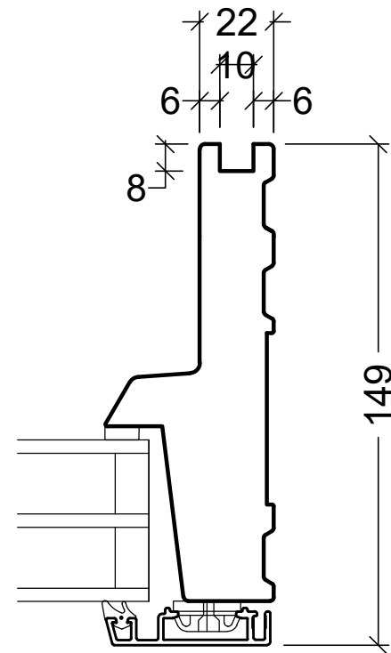
149 mm frame (karm)
